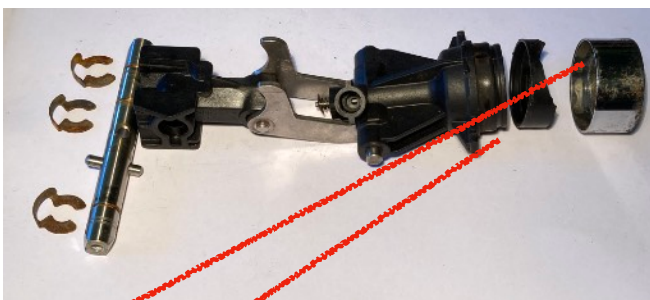
Deze pen schuift uit het plastic blokje en kan dan uit het asje getikt worden
