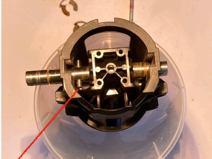
Deze pen schuift uit het plastic blokje en kan dan uit het asje getikt worden
