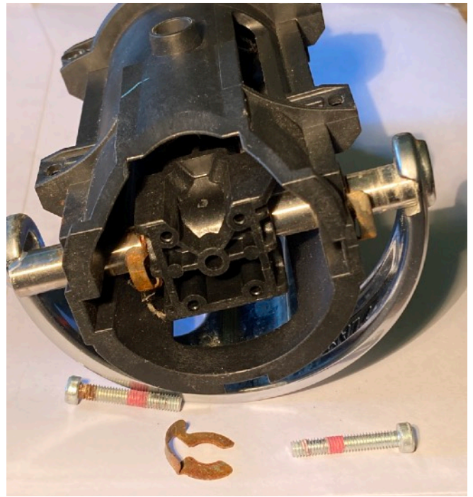
3 asborgringen demonteren en as er uit schuiven. Let op dat kan maar één kant uit die bepaald wordt door de pen op volgende foto
