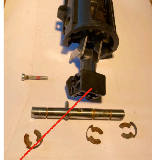
De drijfstang met de verdachte pakking kan nu naar buiten geschoven worden
