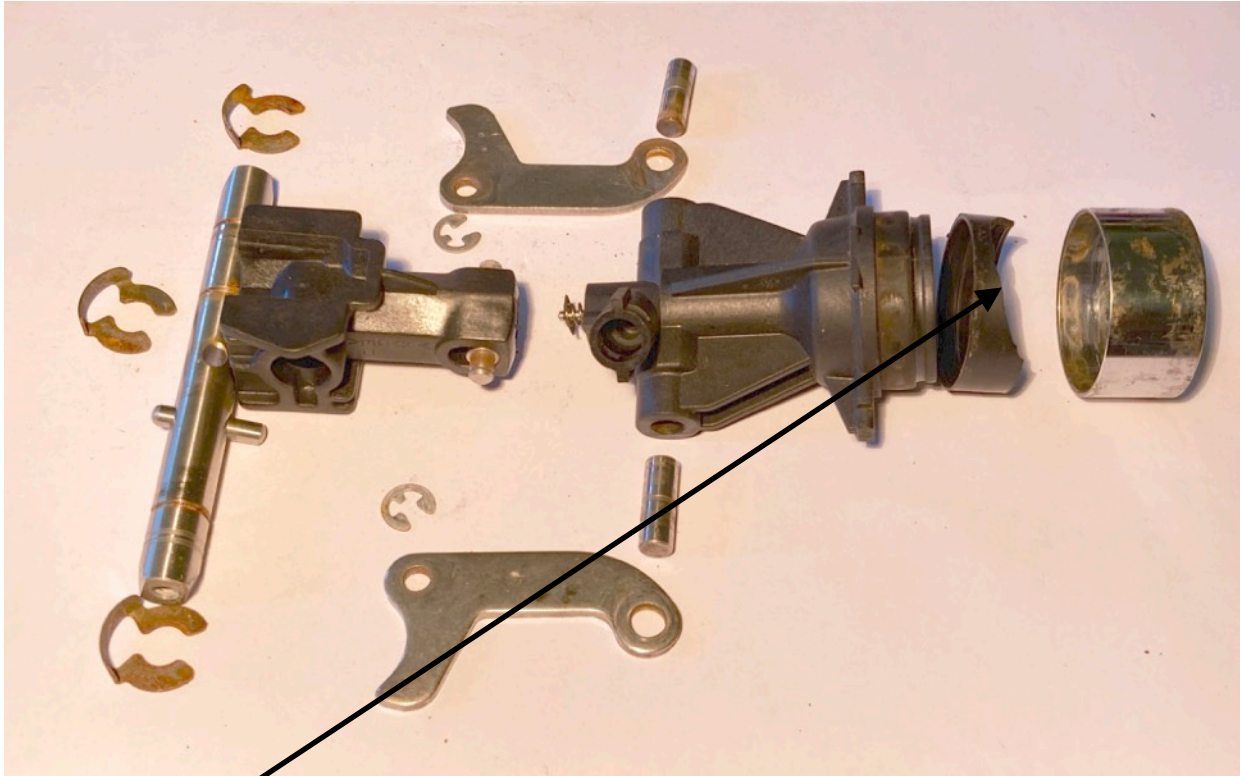
Andere componenten verder los genomen. Duidelijk is te zien welk een grote hap eruit de rubberpakking mist
